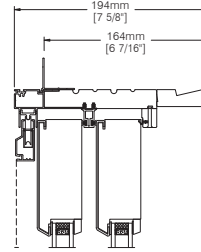
VERTICAL SECTION c/w OPTIONAL 164mm JAMB LINER
