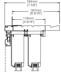
VERTICAL SECTION c/w OPTIONAL 167mm JAMB LINER
